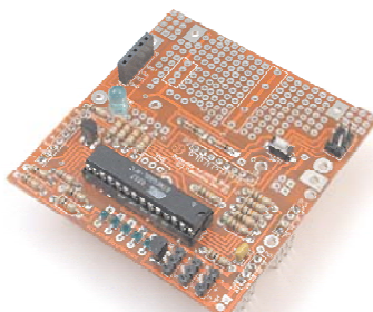
Atmel Mega 8
